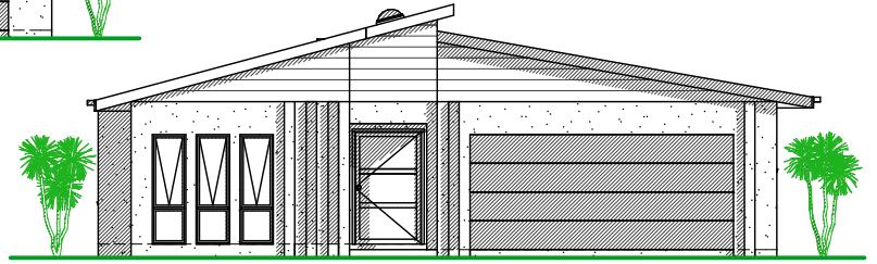
ELEVATION - V2
