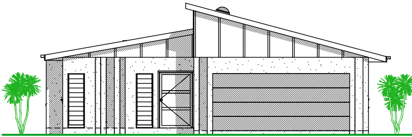
ELEVATION - V1
