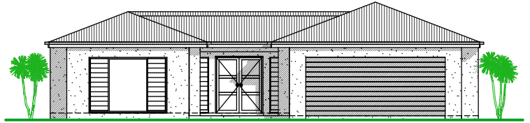
ELEVATION 2
