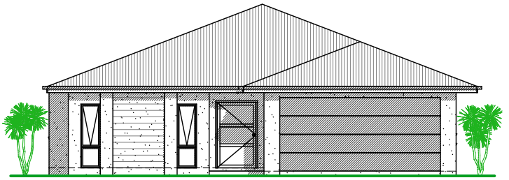
ELEVATION - V2
