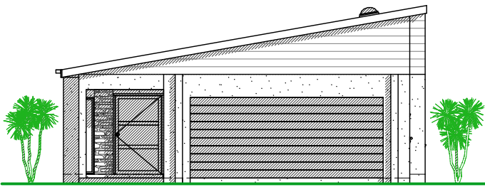
ELEVATION - V1
