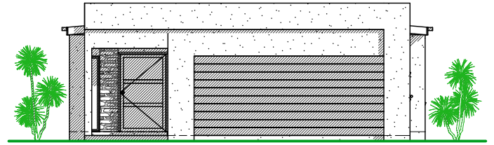
ELEVATION - V2
